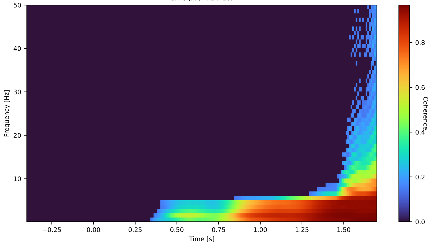
dPFC (F7) - PE (P20)
